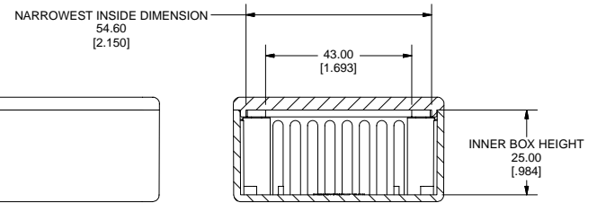
SECTION D-D SCALE 1 : 1
