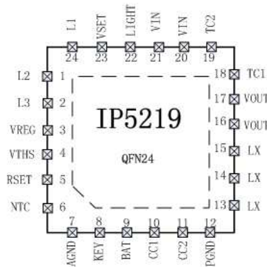
图 2 IP5219 引脚图
